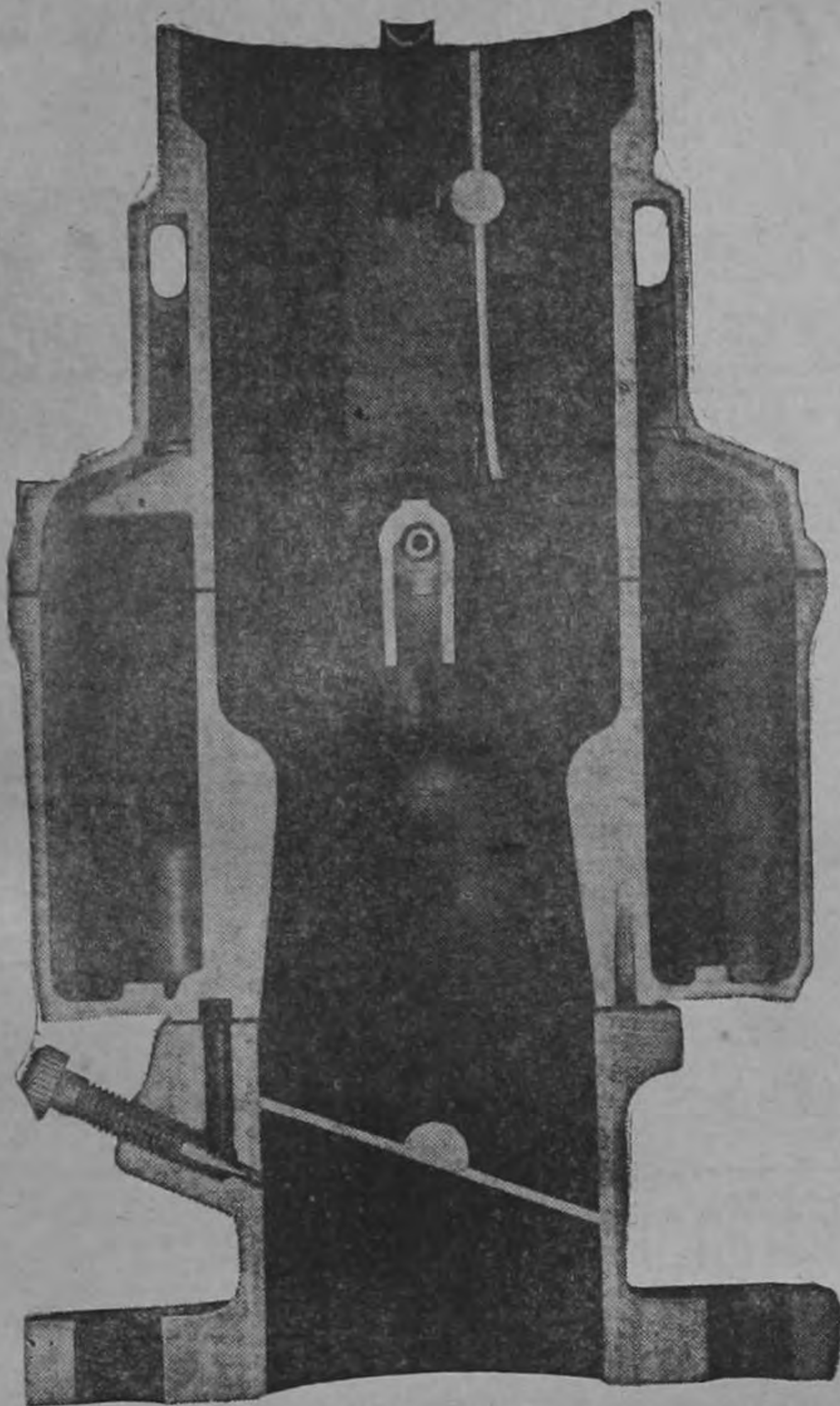
Corte seccional de un carburador mostrando depósitos de goma y carbón.
