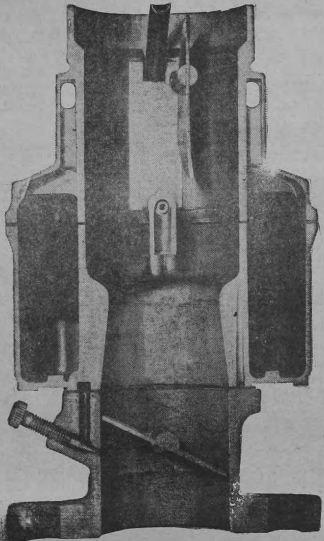
Corte de un carburador limpio.
